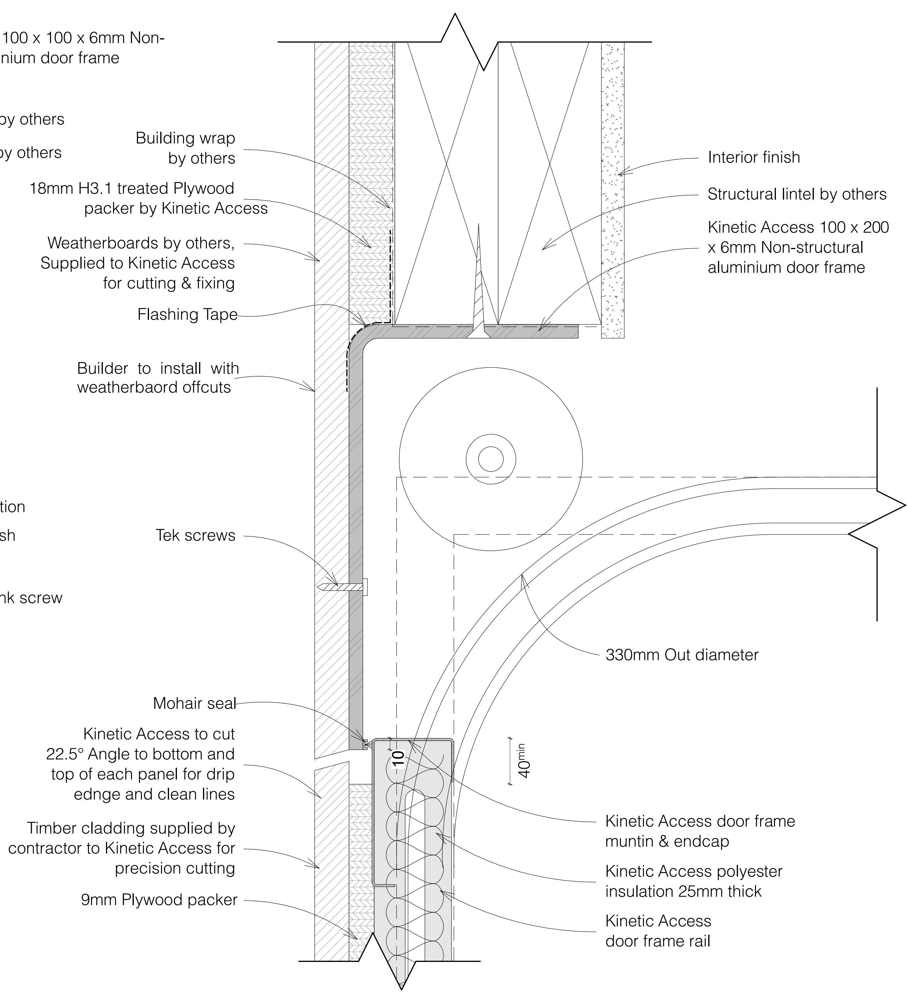
2 Garage Door Head Detail 1 : 2
