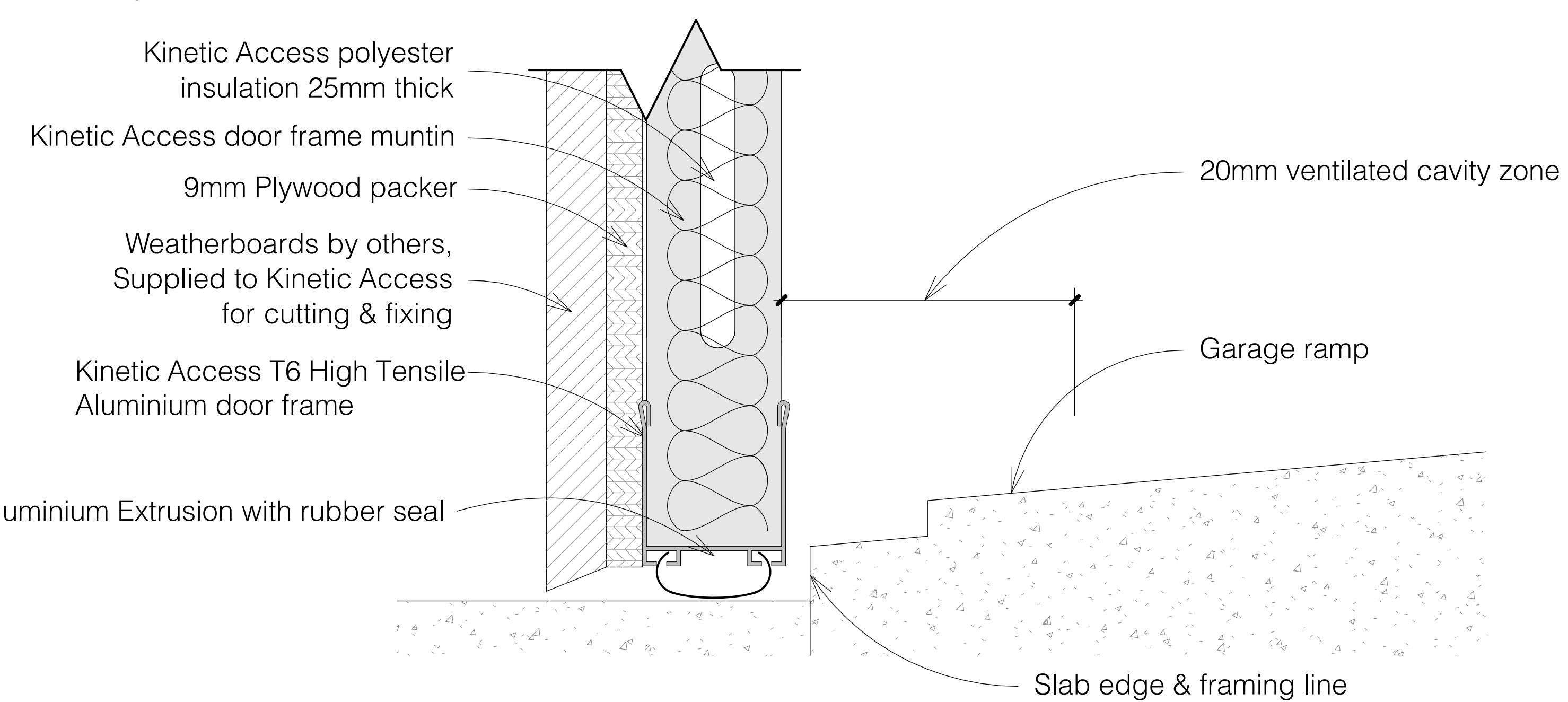
3 Garage Door Foundation Detail 1 : 2
